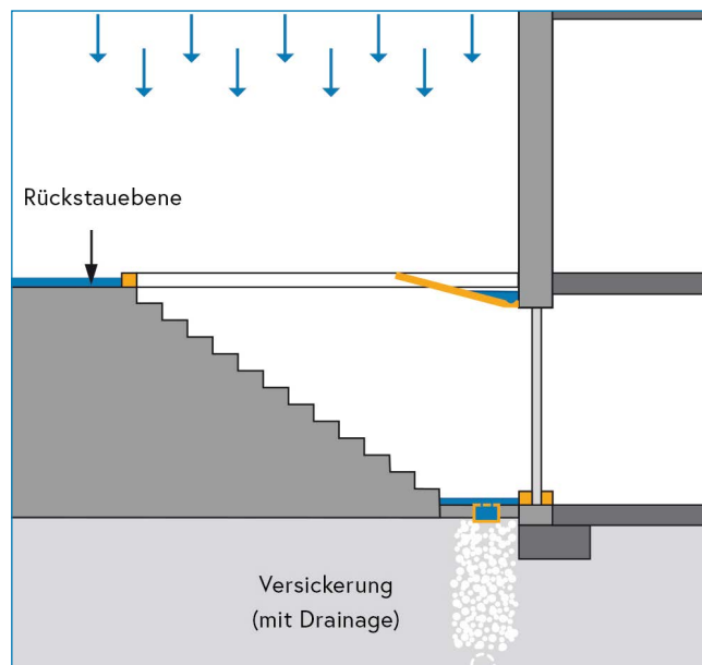
Abbildung 28: Richtig geschützte Kellertreppe (Schemaskizze).
