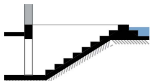
Abbildung 59: Nachträglich durch Aufmauerung geschützter Kellertreppenzugang.
