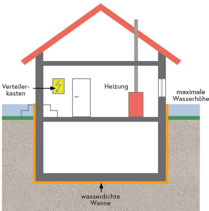
Abbildung 54: Hochwassersichere Installation von Stromverteiler und Heizanlage. Auf Ölheizungen sollte in hochwassergefährdeten Gebieten generell verzichtet werden.
