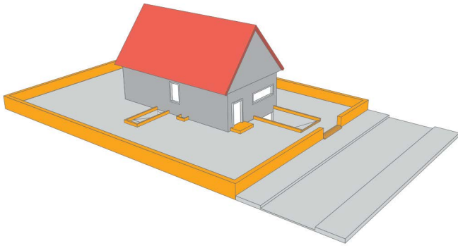
Abbildung 22: Aufmauerungen können an vielen Stellen Wassereintritte verhindern.
