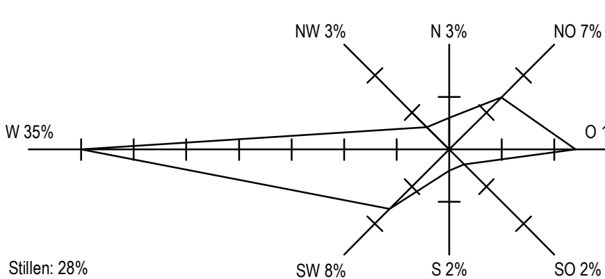
Diagramm der Windrichtungshäufigkeit
